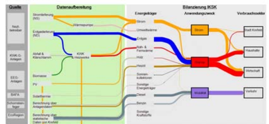
IKSK Stadt Krefeld - Energiebilanz 2017 Datenaufbereitung
